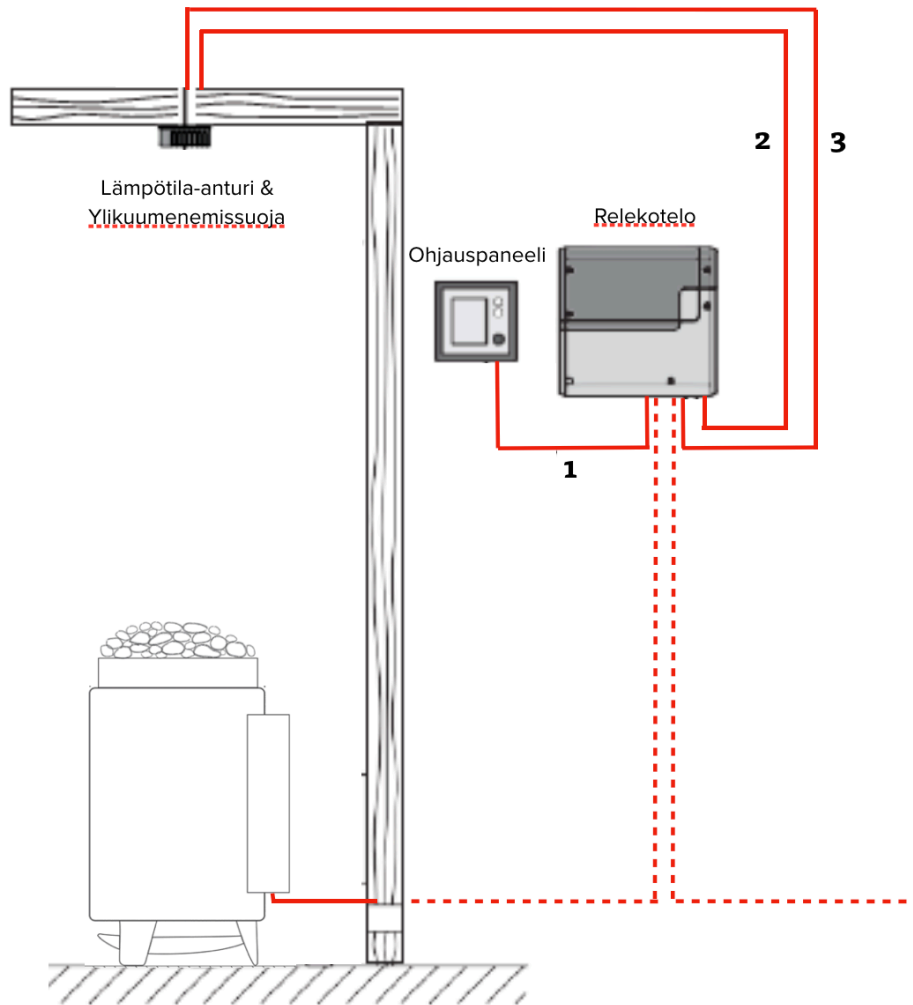
Kuva: VETO kiukaan kanssa yhteensopivan erillisen ohjauskeskuksen johdotus (poislukien Econ D2).
